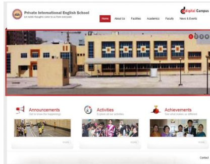
Web Portal
